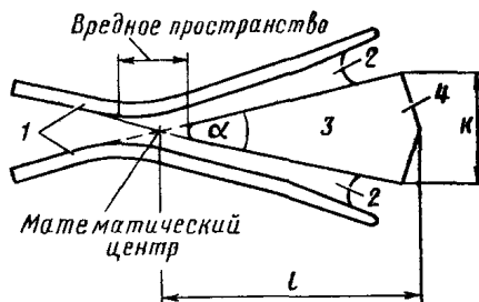
1 — усовики; 2 — желоба; 3 — сердечник; 4 — хвост крестовины Рисунок 41. Схема крестовины
