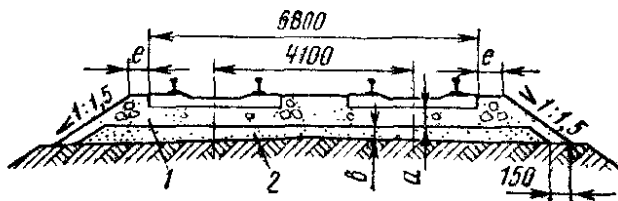
Рисунок 26. Поперечный профиль балластной призмы для главных путей двухпутной линии
