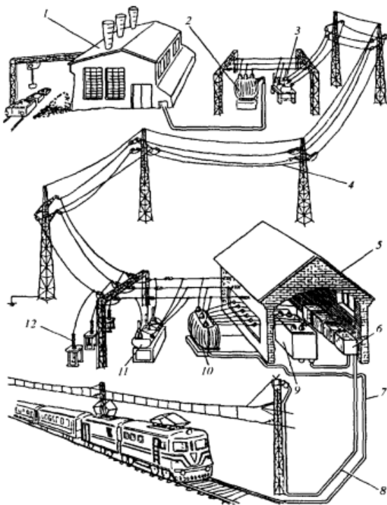
1 — электростанция; 2— повышающий трансформатор; 3 — высоковольтный выключатель; 4 — линия электропередачи; 5 — тяговая подстанция; 6 — блок быстродействующих выключателей и разъединителей; 7 — отсасывающая линия; 8 — питающая линия; 9 — выпрямитель; 10—тяговый трансформатор; 11 — высоковольтный выключатель; 12 — разрядник
