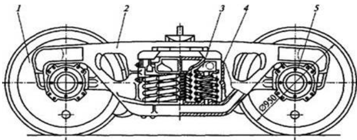
Рисунок 73. Тележка пассажирского вагона КВЗ-ЦНИИ
