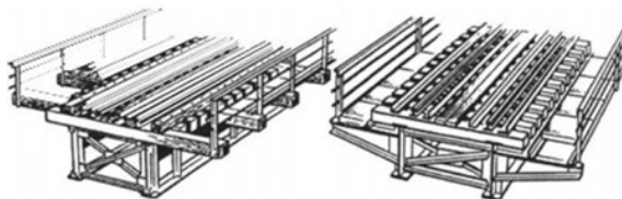
Рисунок 39. Конструкции пути на постоянных мостах
