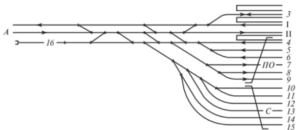
ПО — приемоотправочный парк; С — сортировочный парк Рисунок 80. Схема стрелочной горловины станции
