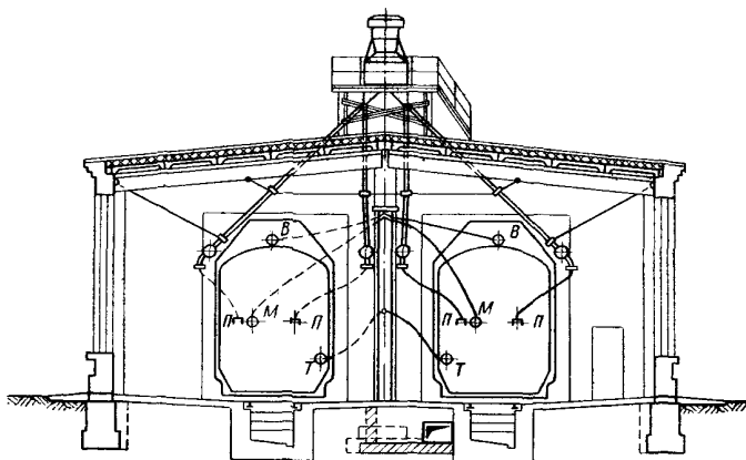
Т, П, М, В — гибкие шланги для подачи соответственно топлива, песка, масла, воды Рисунок 76. Схема расположения экипировочных устройств для тепловозов в утепленном помещении:
