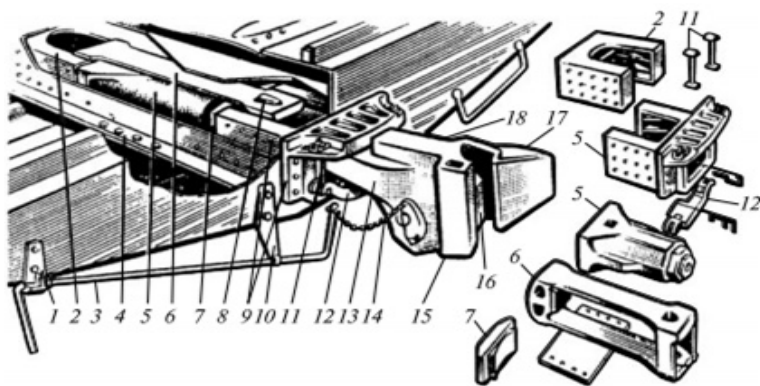
1 — кронштейн; 2 — задний упор; 3 — расцепкой рычаг; 4 — поддерживающая планка; 5 — поглощающий аппарат; 6 — тяговый хомут; 7 — упорная плита; 8 — клин; 9 — передний упор и ударная розетка; 10— державка; 11 — маятниковая подвеска; 12— центрирующая балка; 13 — корпус автосцепки; 14 — цепь; 15 — малый зуб; 16 — замок; 17 — большой зуб; 18 — упор Рисунок 75. Автосцепное устройство вагона
