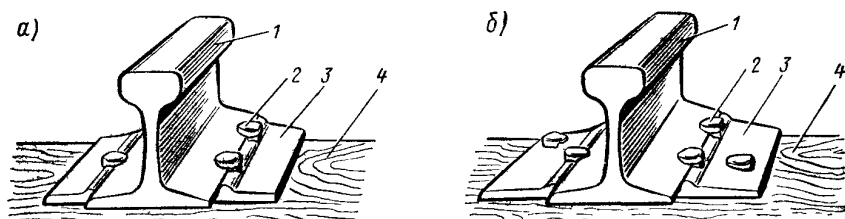
а — нераздельное; б — смешанное; 1 — рельс; 2 — костыль; 3 — подкладка; 4 — шпала
