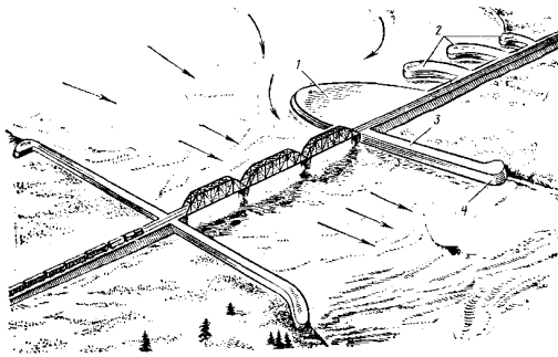
1 — грушевидная дамба; 2 — траверсы; 3 — шпоровидная дамба; 4 — голова дамбы
