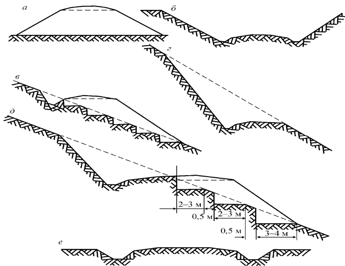
а – насыпь, б-выемка, г- полувыемка, д- полунасыпь-полувыемка, е - нулевое место Рисунок 9. Поперечные профили земляного полотна
