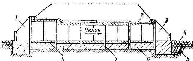
Рисунок 22. Продольный разрез трубы
